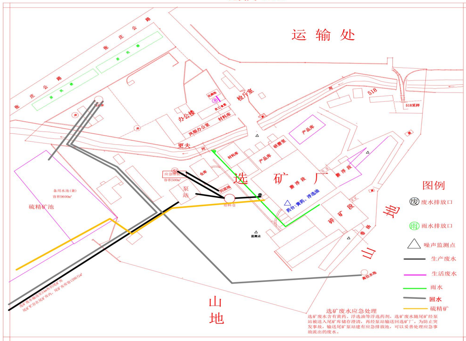
图 4.2.5-2 丹东青城子矿业有限公司（选矿厂）管线布置图
